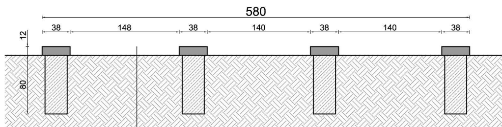
przekrój A-A
