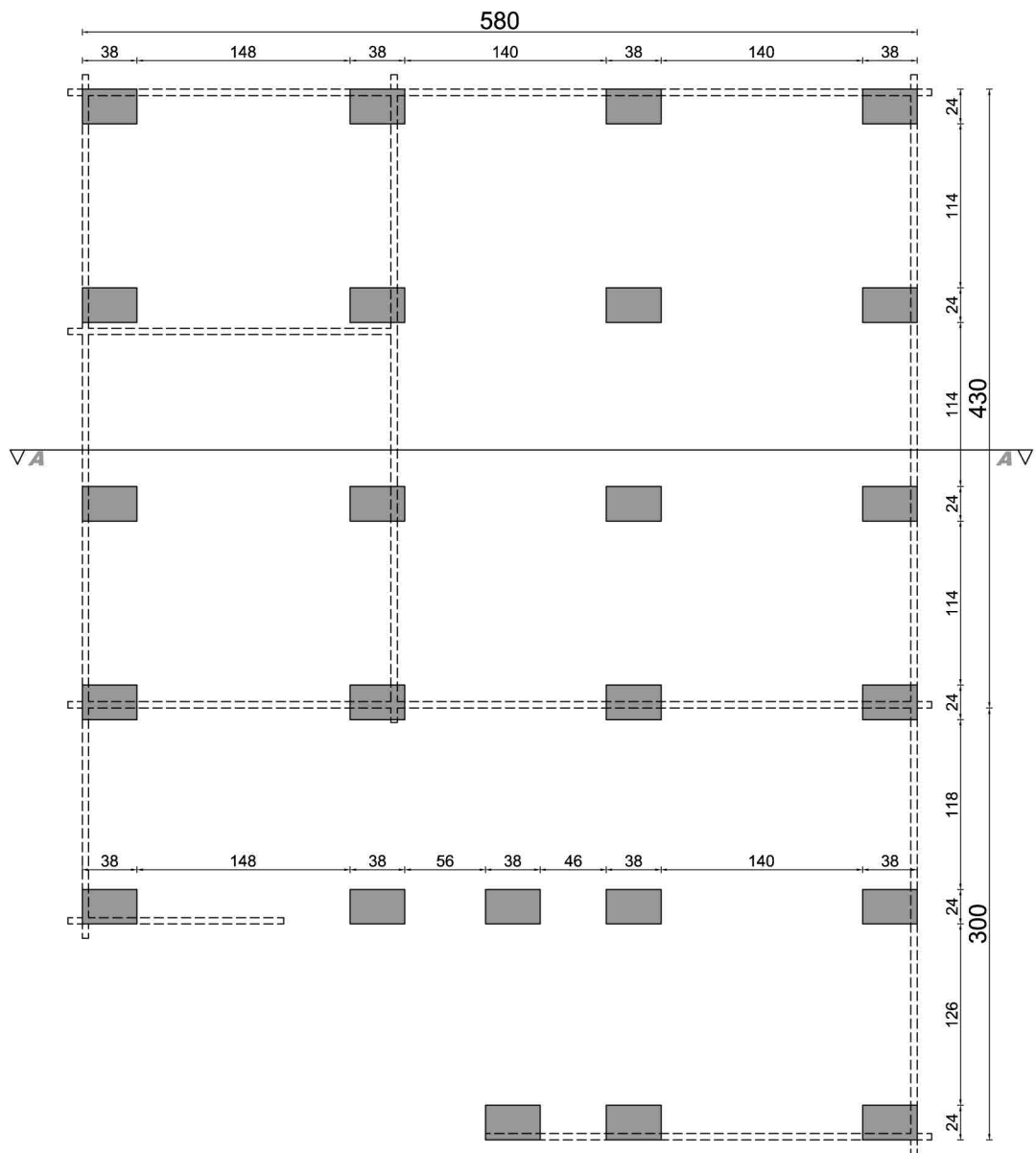
rzut fundamentów
