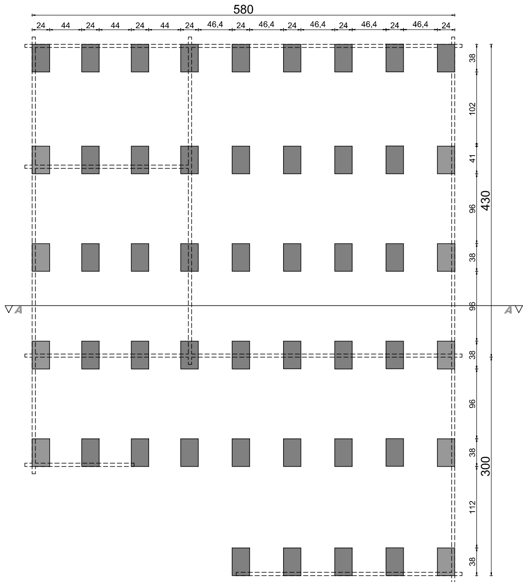
rzut fundamentów
