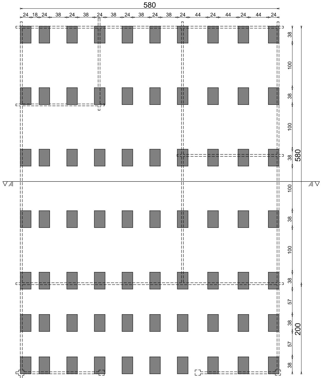
rzut fundamentów
