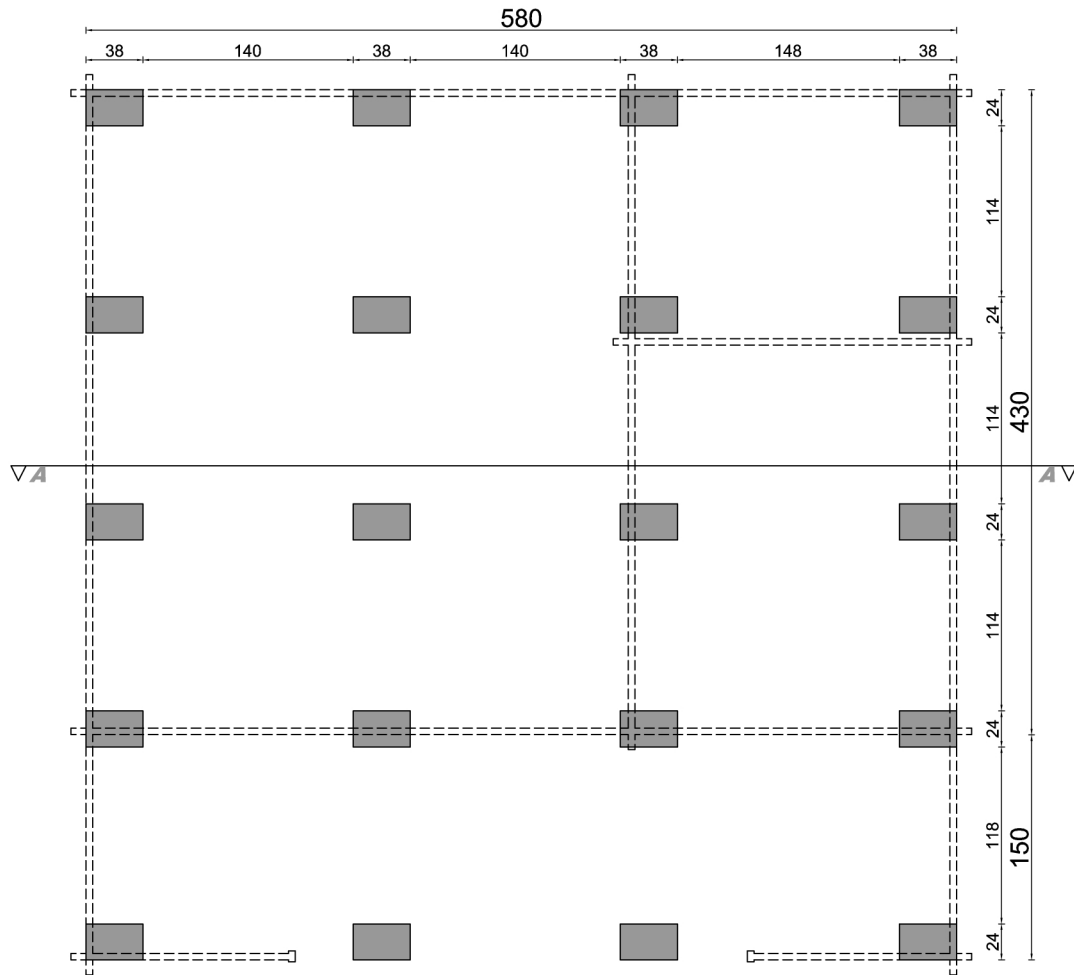
rzut fundamentów
