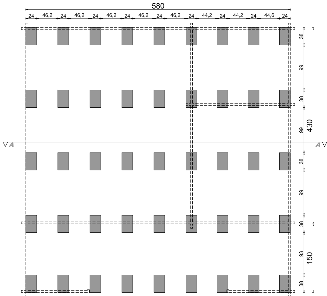
rzut fundamentów
