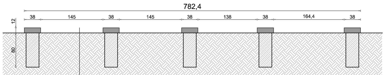
przekrój A-A
