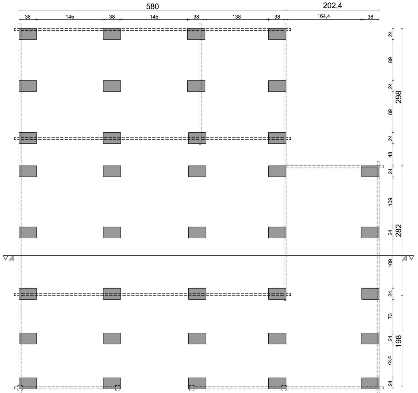
rzut fundamentów
