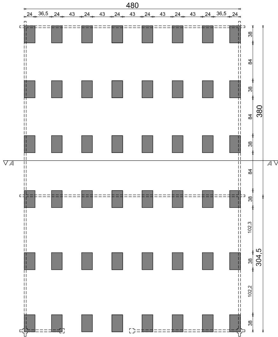
rzut fundamentów
