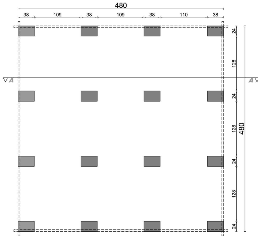
rzut fundamentów
