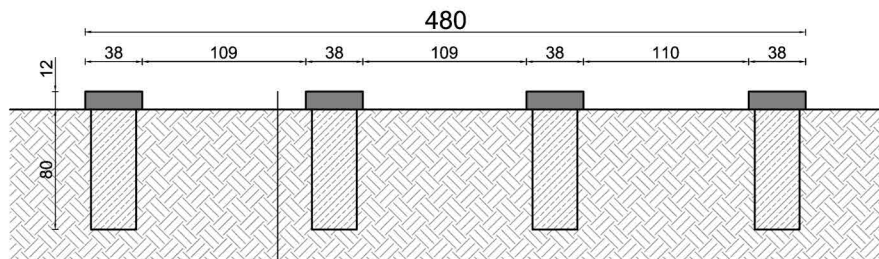
przekrój A-A
