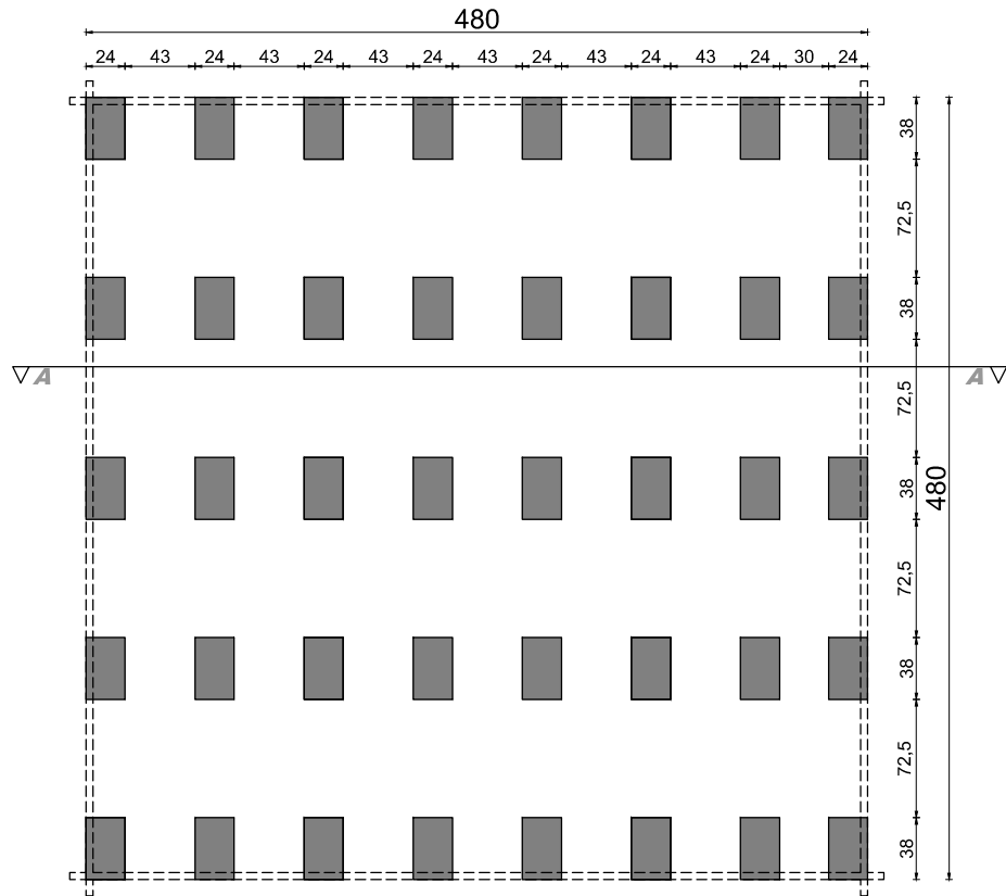
rzut fundamentów
