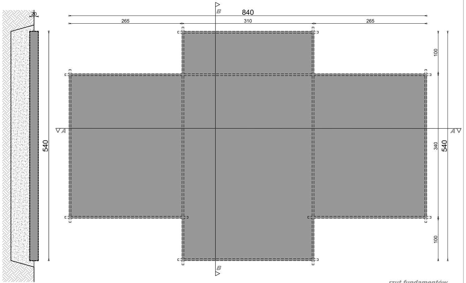
rzut fundamentów
