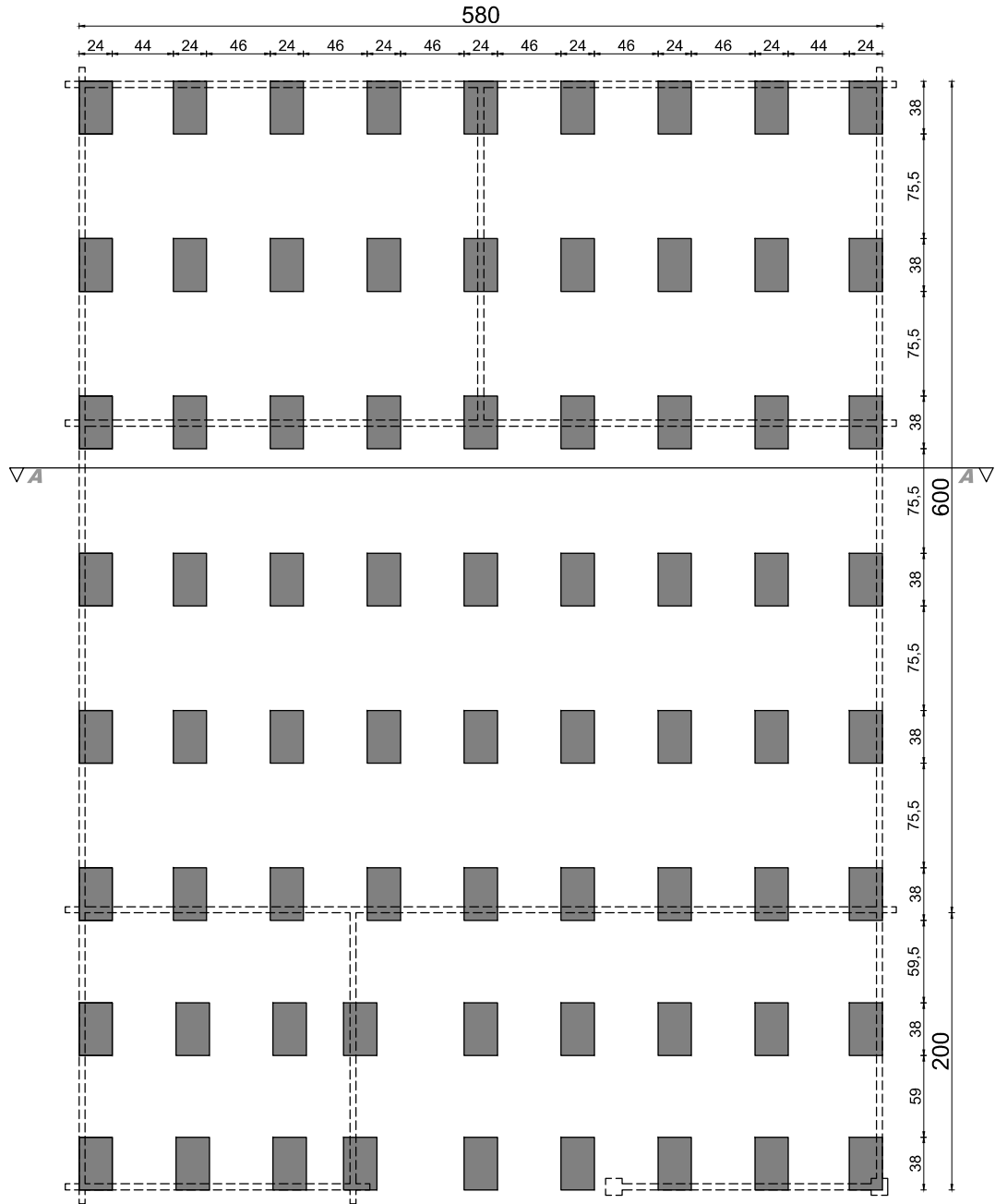
rzut fundamentów
