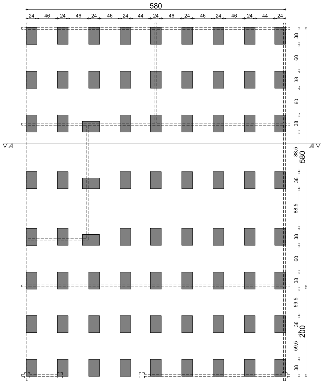
rzut fundamentów
