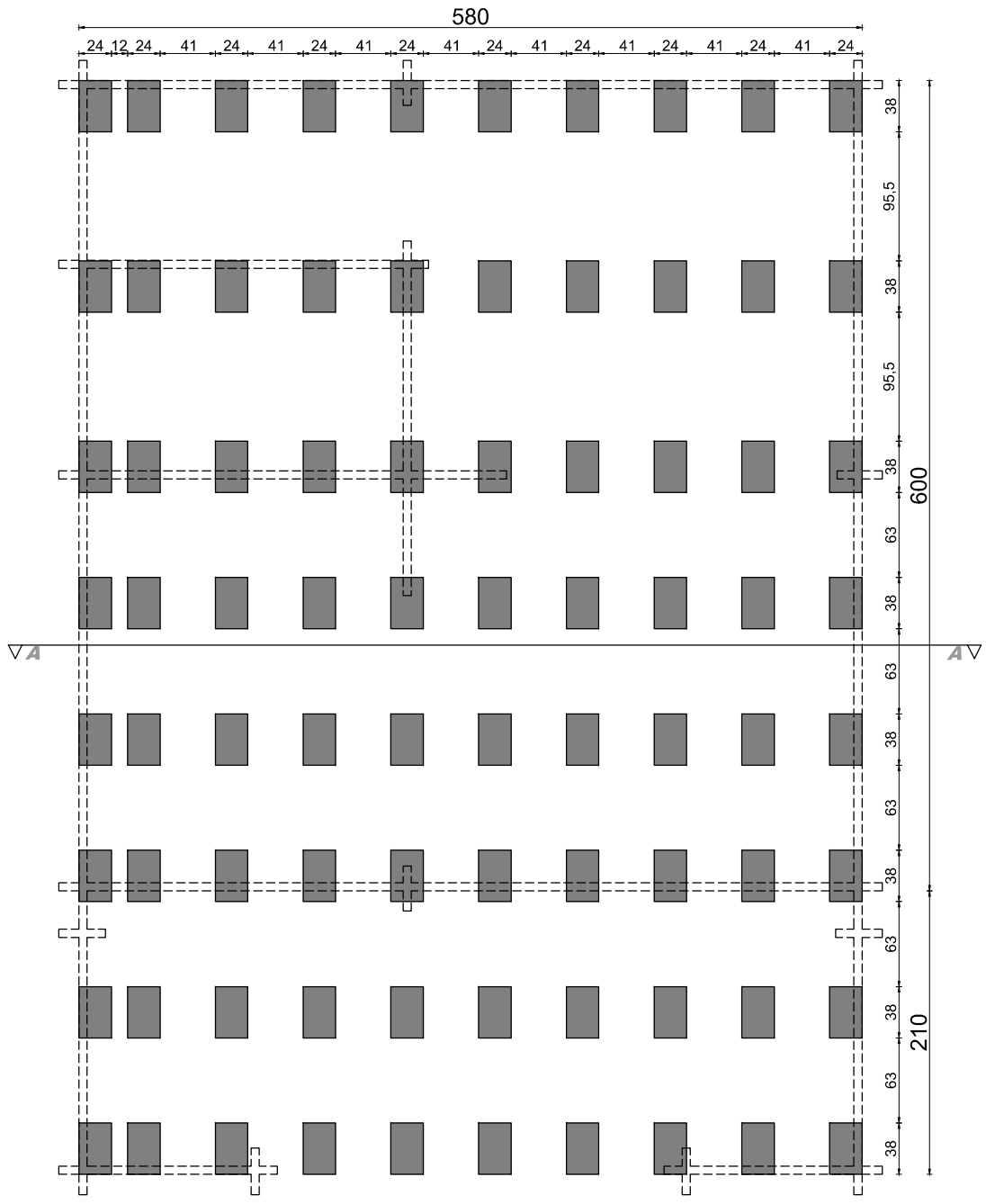
rzut fundamentów
