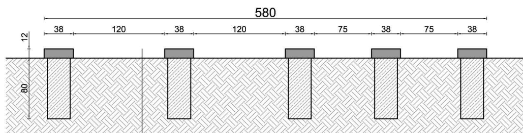
przekrój A-A
