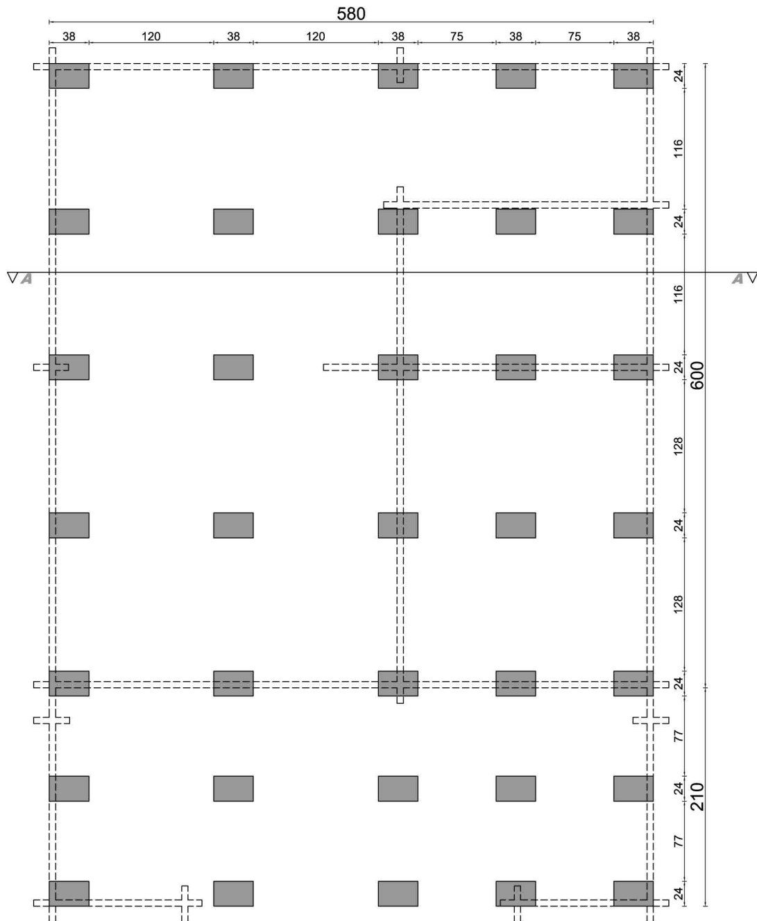
rzut fundamentów
