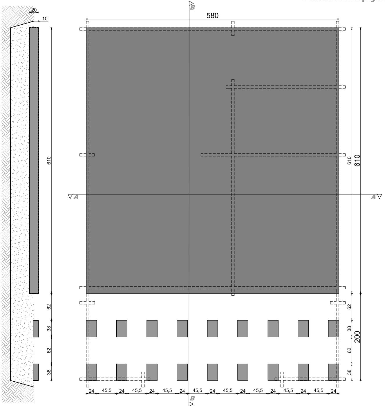
rzut fundamentów
