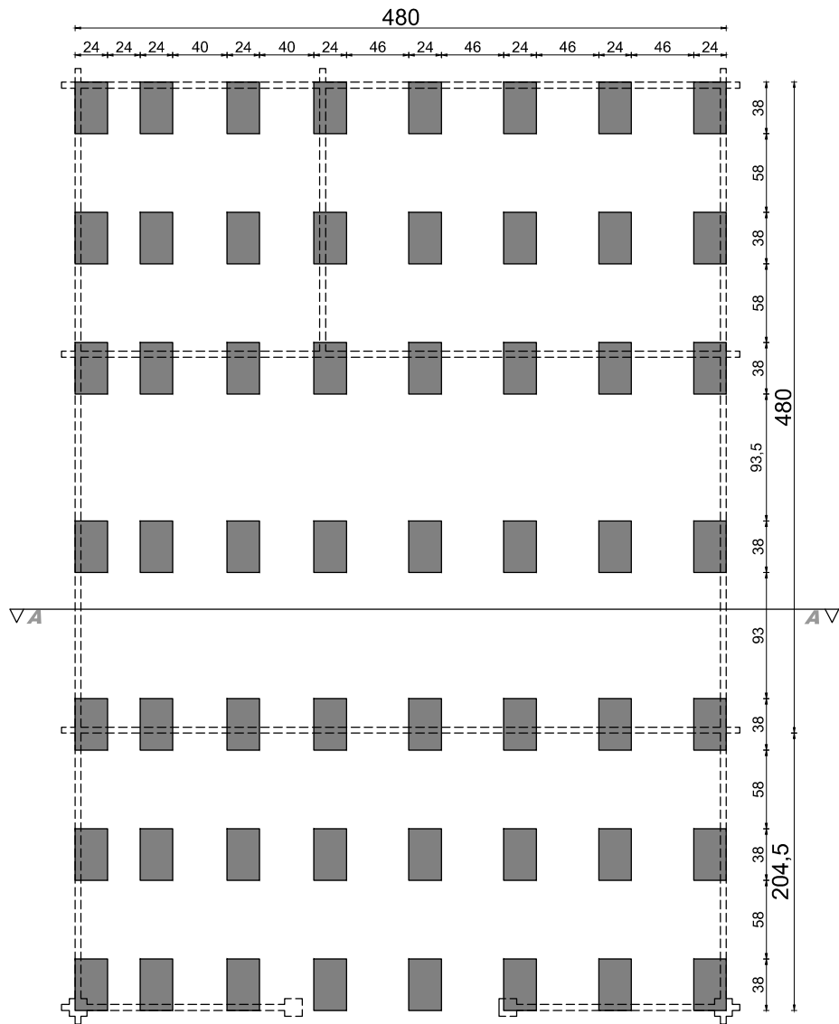
rzut fundamentów
