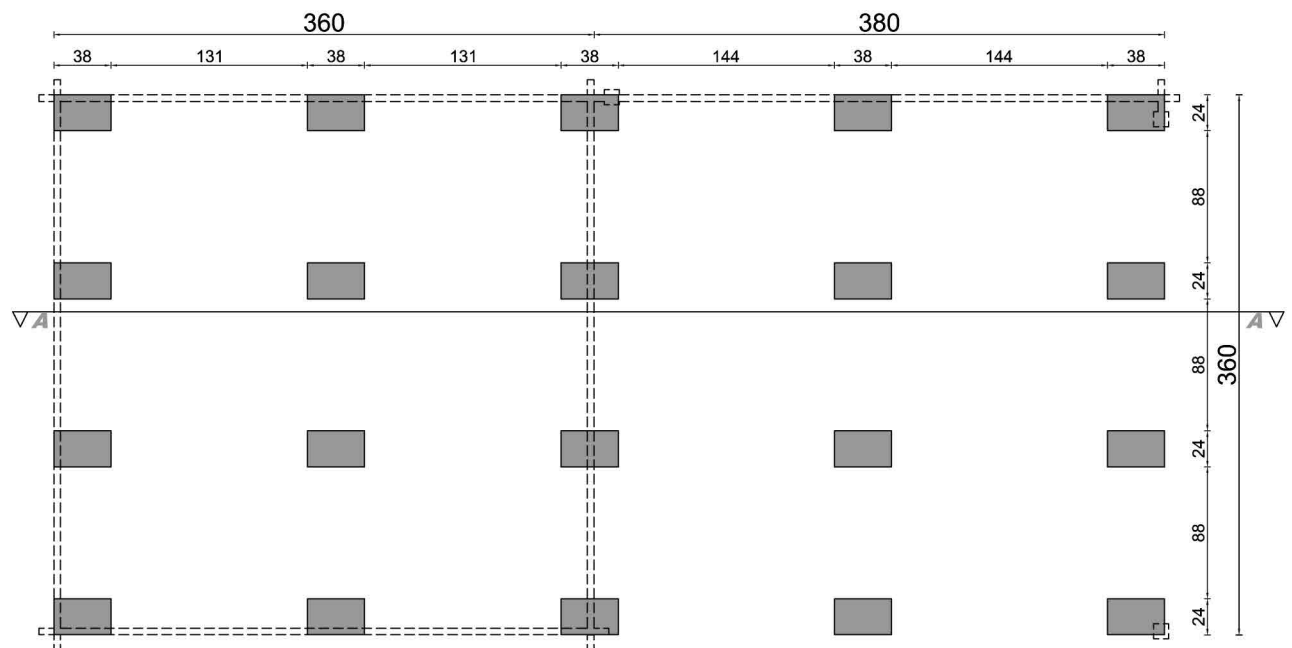
rzut fundamentów
