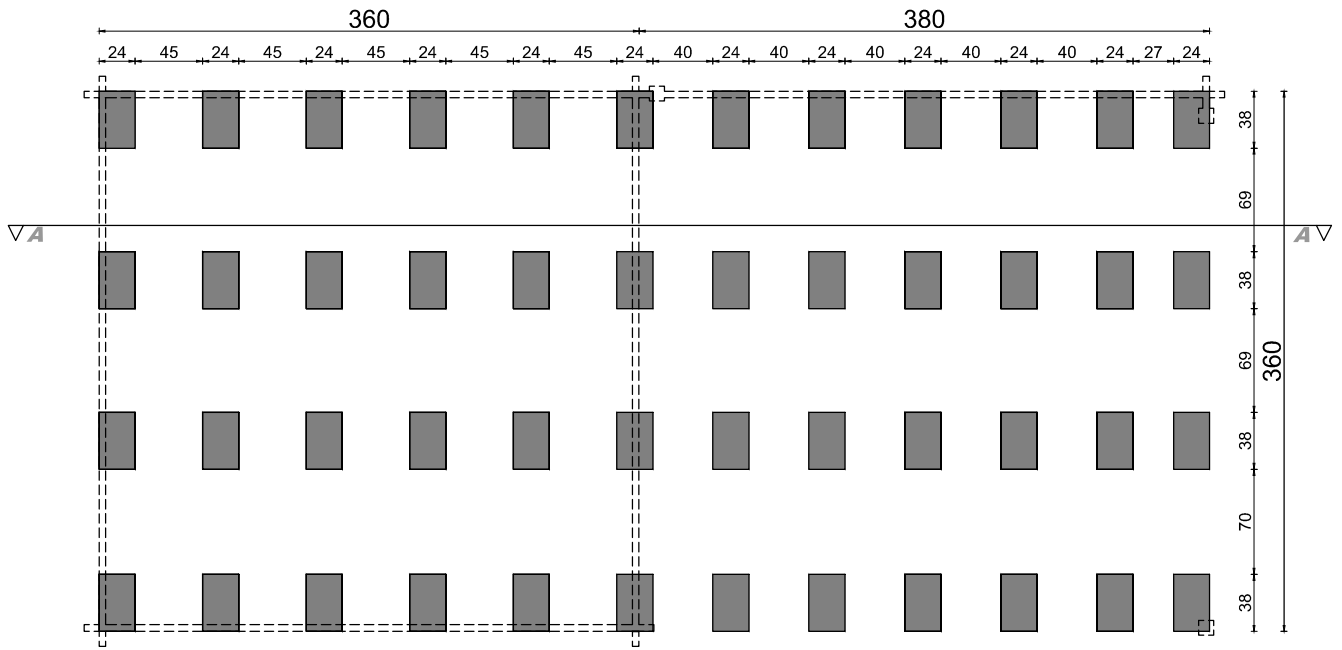
rzut fundamentów
