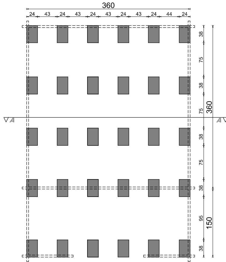
rzut fundamentów
