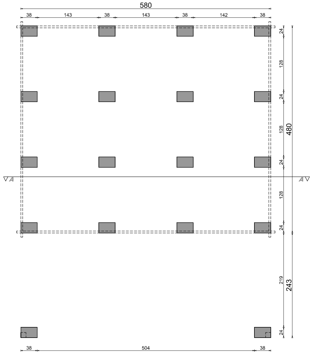
rzut fundamentów
