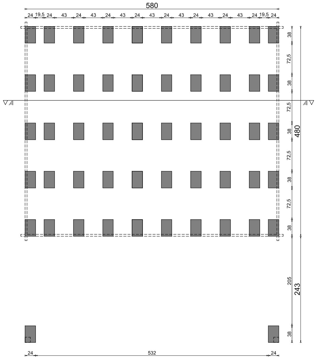
rzut fundamentów
