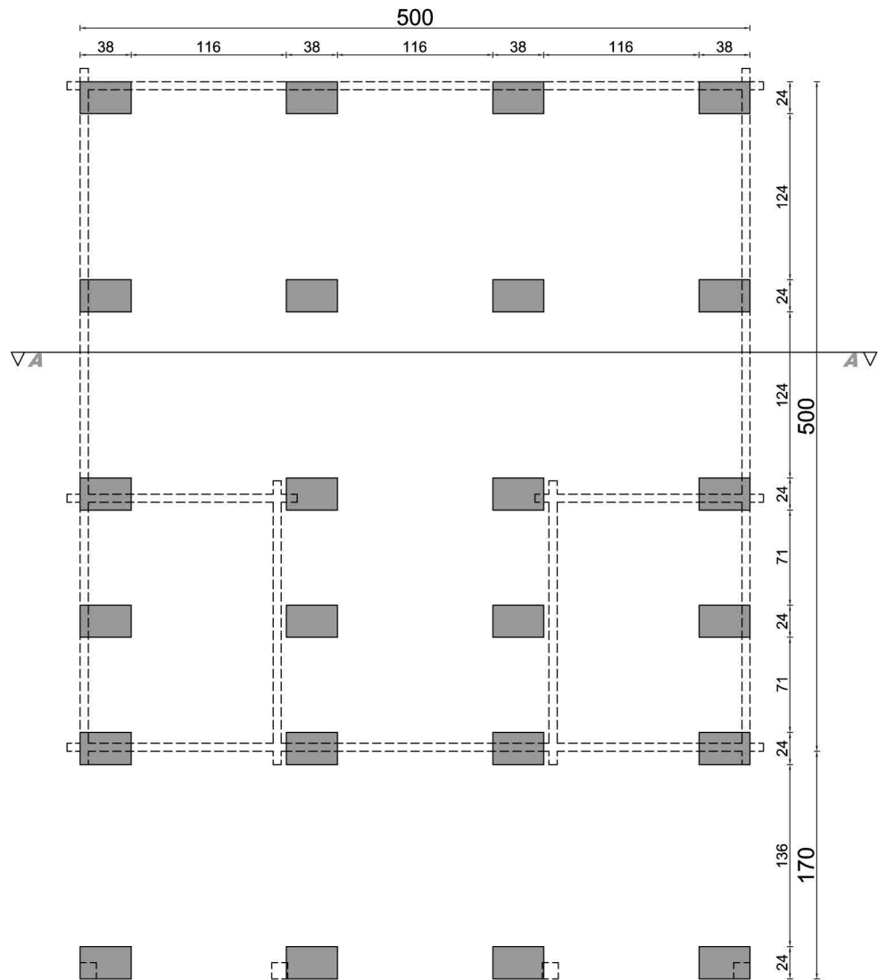
rzut fundamentów
