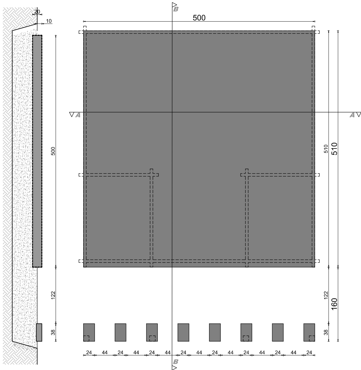
rzut fundamentów
