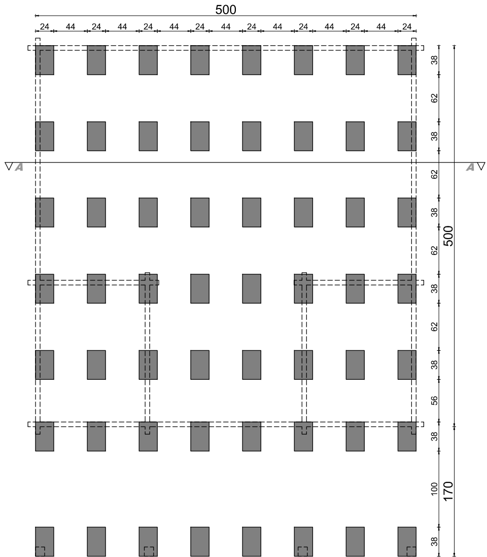
rzut fundamentów
