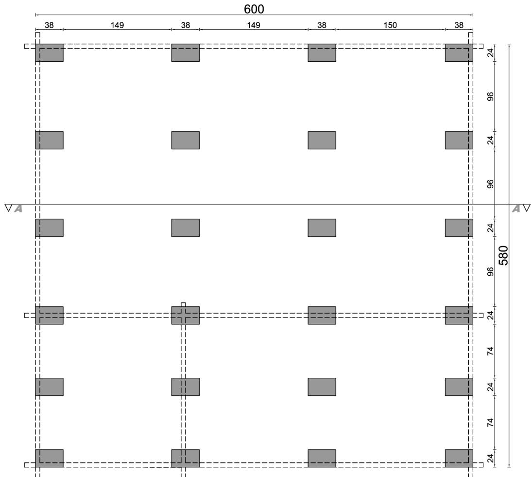
rzut fundamentów
