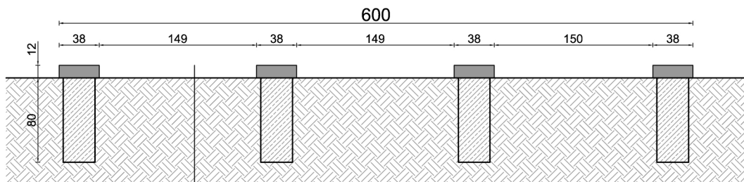
przekrój A-A
