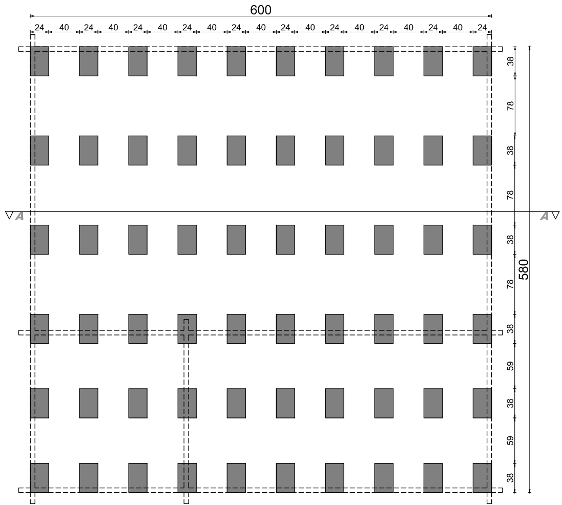
rzut fundamentów
