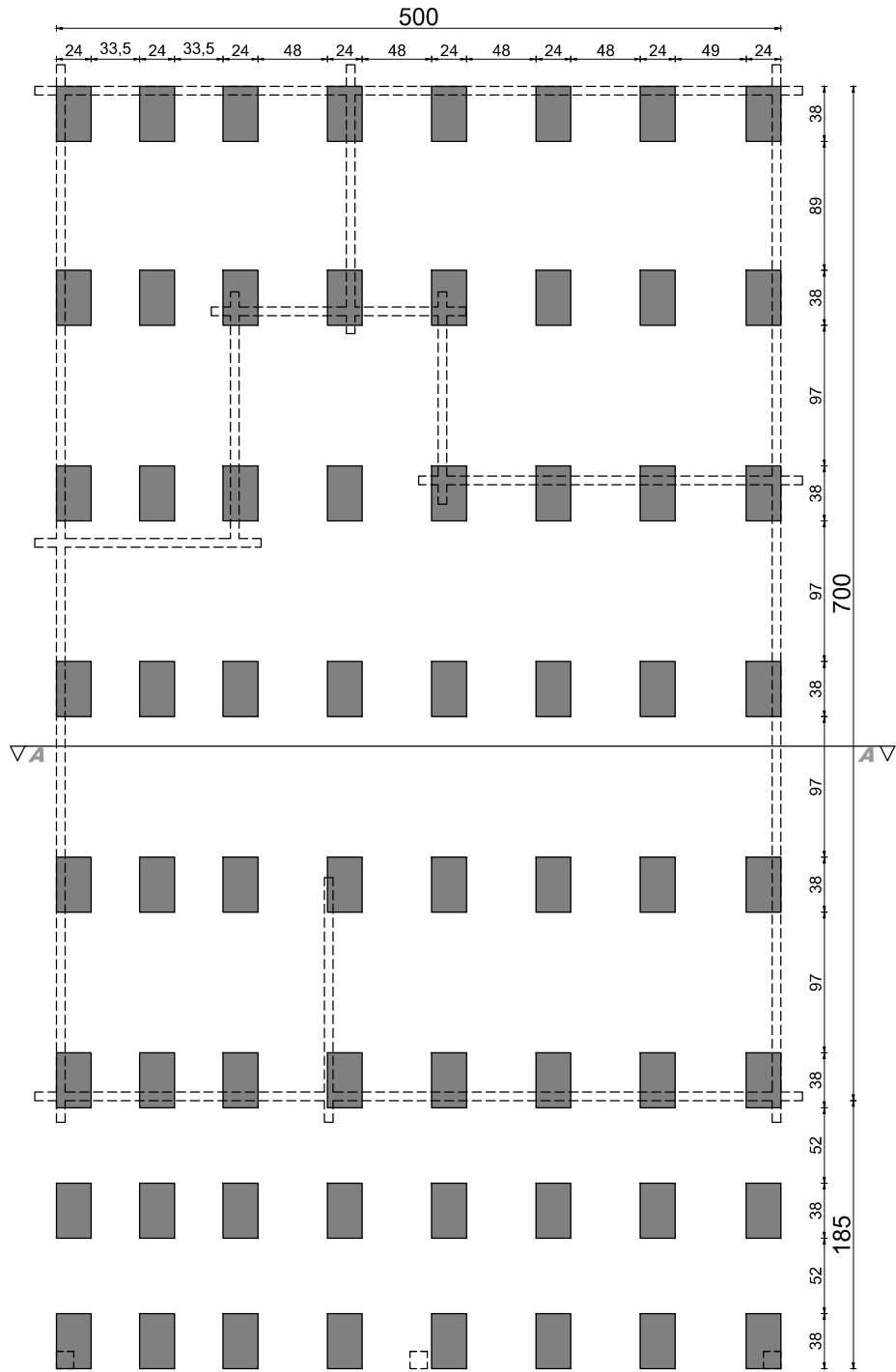
rzut fundamentów
