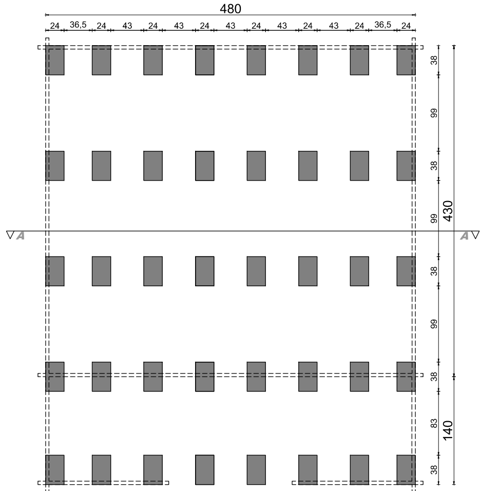
rzut fundamentów
