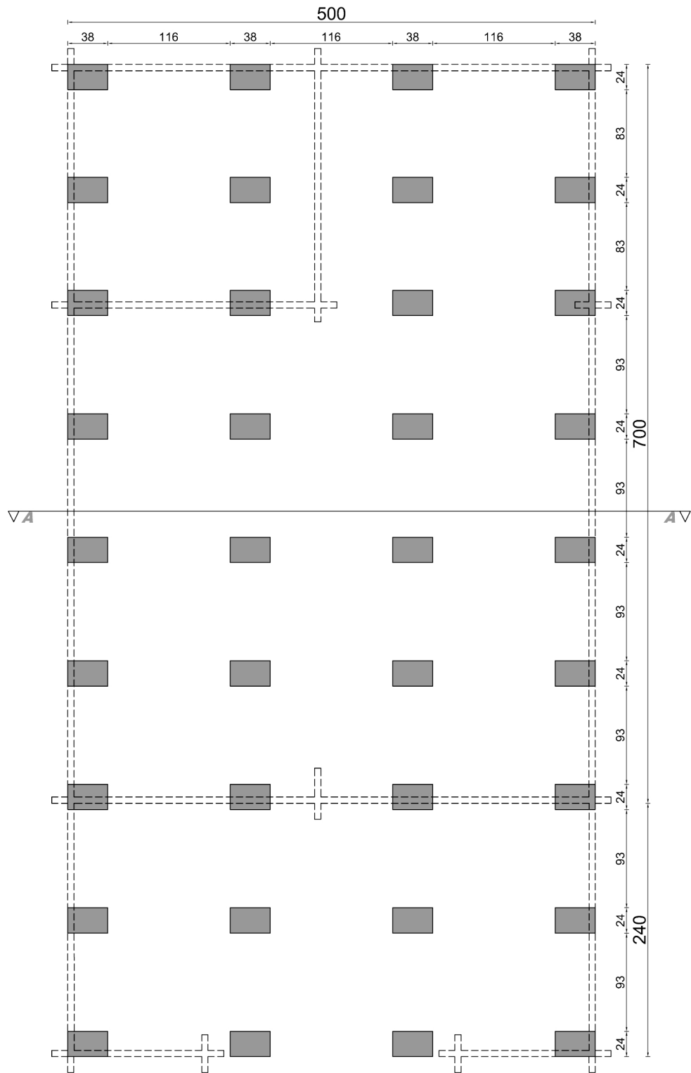
rzut fundamentów
