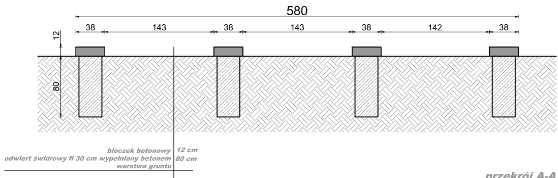
przekrój A-A
