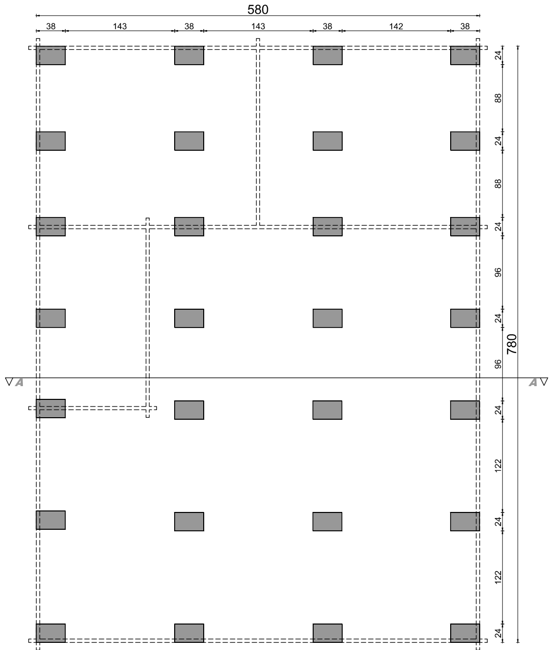
rzut fundamentów
