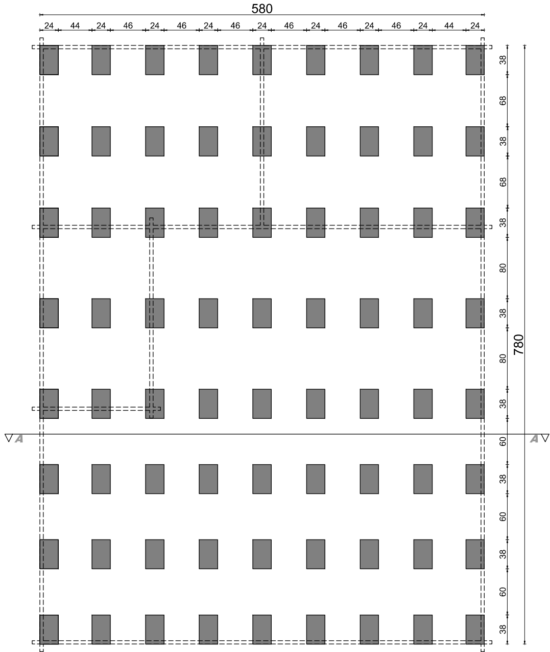
rzut fundamentów
