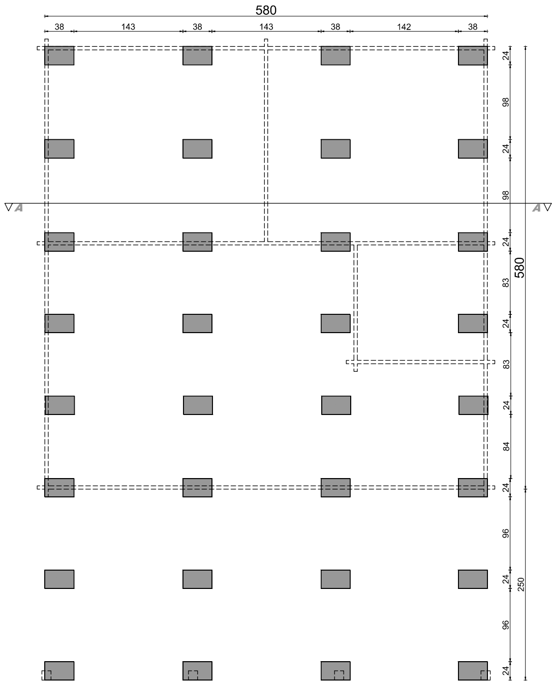
rzut fundamentów
