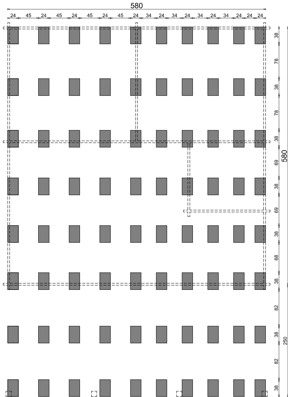
rzut fundamentów
