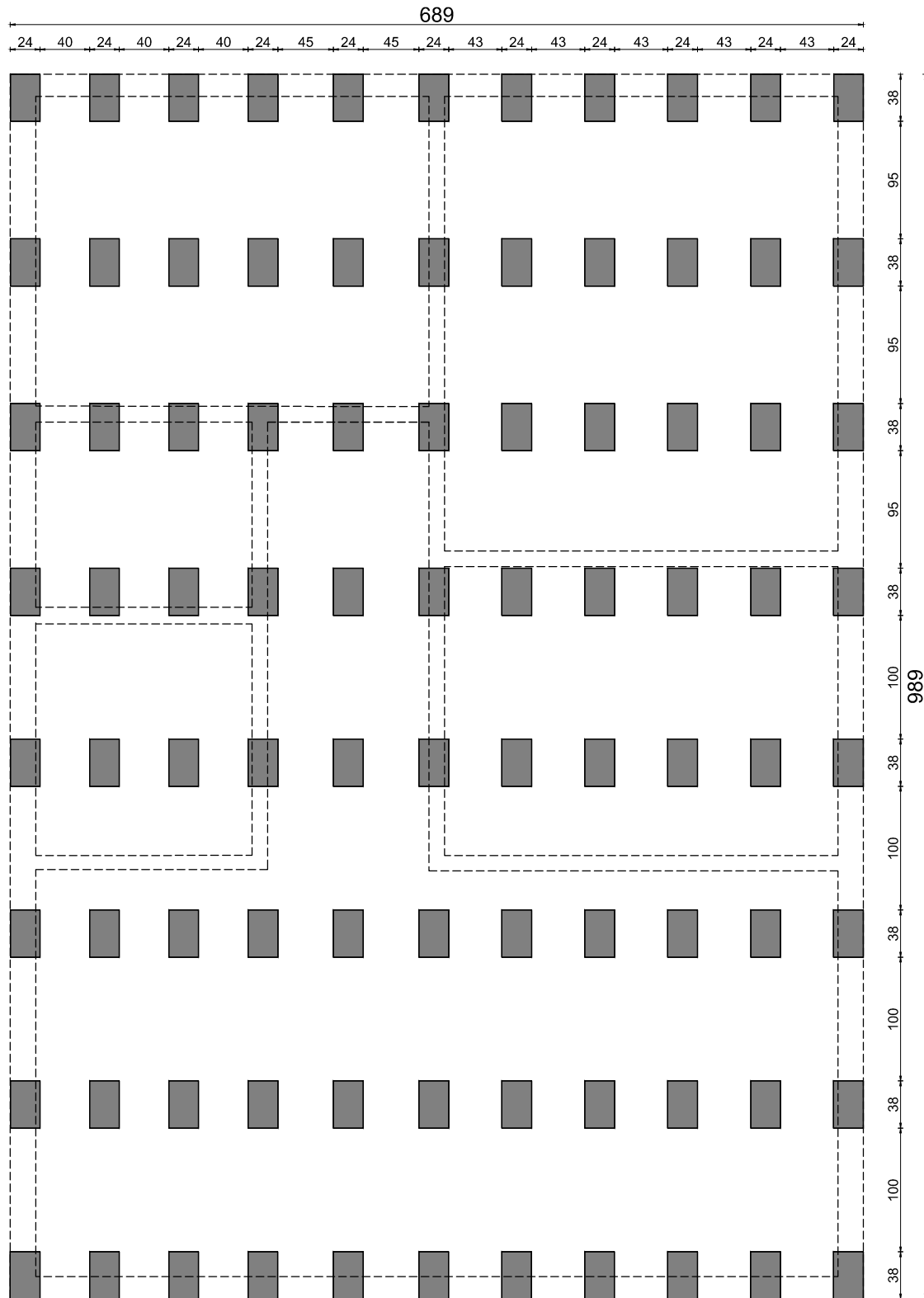
rzut fundamentów
