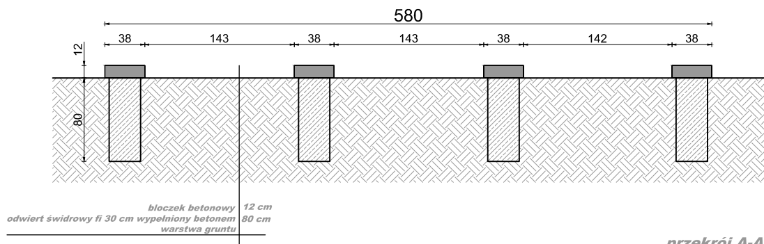
przekrój A-A
