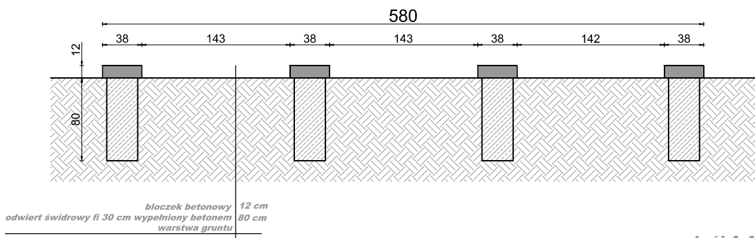
przekrój A-A
