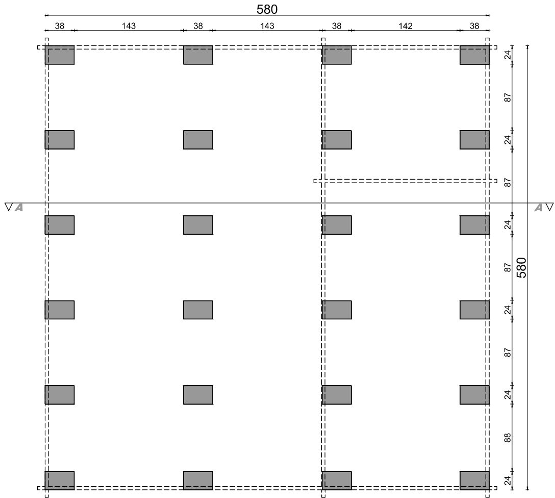
rzut fundamentów
