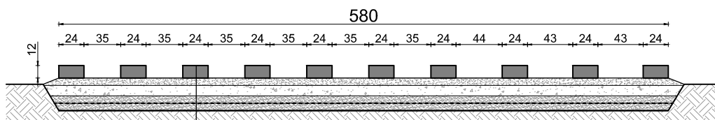
przekrój A-A
