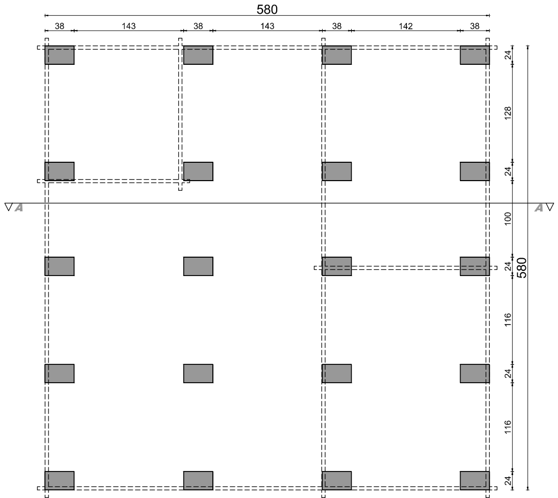
rzut fundamentów
