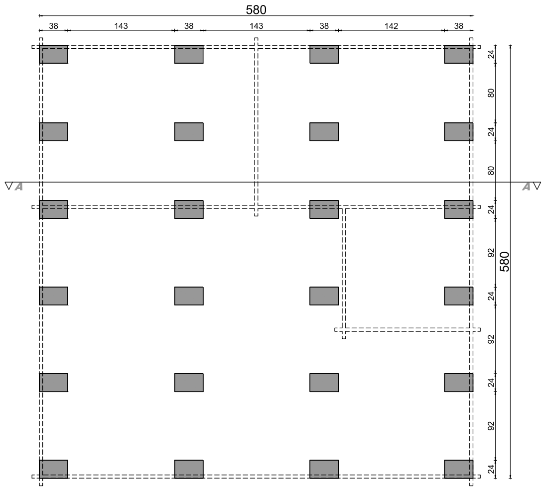
rzut fundamentów
