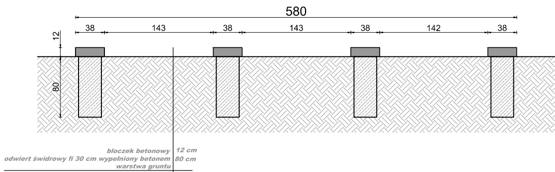
przekrój A-A
