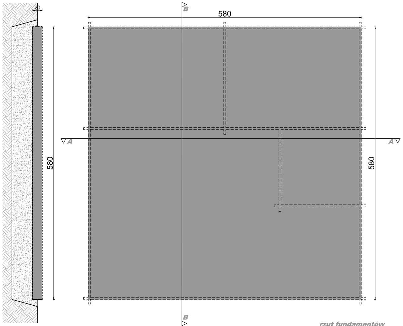
przekrój B-B
