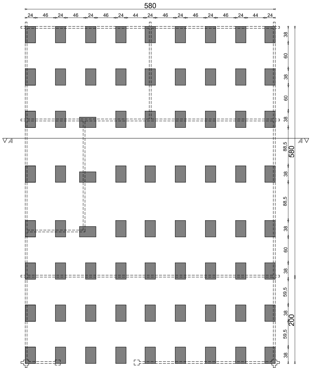
rzut fundamentów
