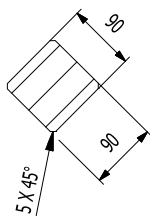
H-H ( 1 : 10 )
