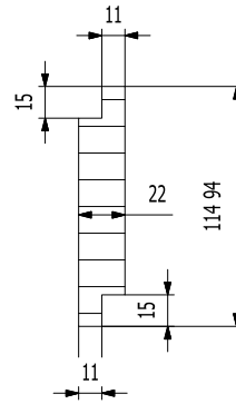
R-R ( 1 : 4 )
